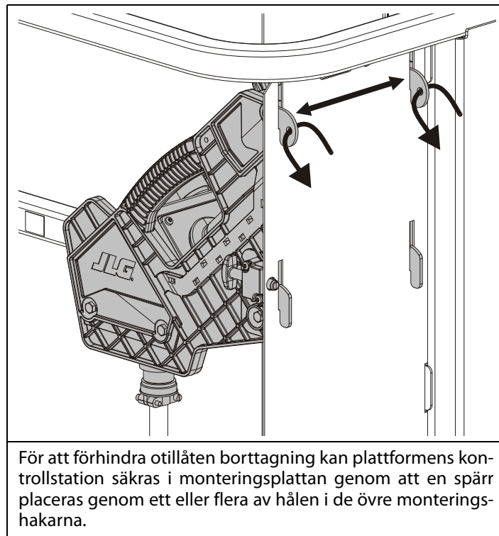
Fig. 4-13. Fastsättning av manöverpanelen i plattformen
