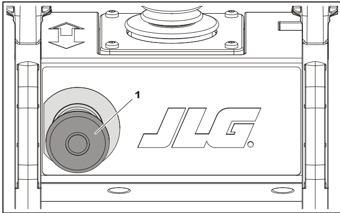
Fig. 4-5. Plattformspanel – nödstoppskontakt
