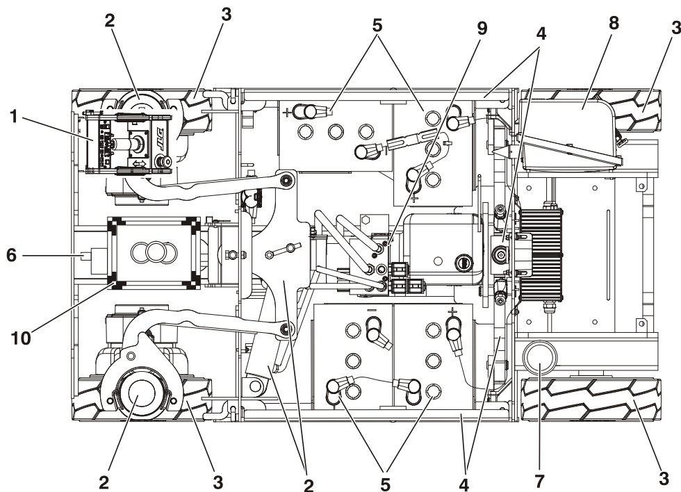
Fig. 2-1. Daglig rundvandningsinspektion (genomskäring ovanifrån)
