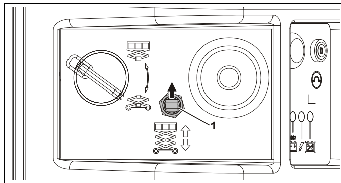
Fig. 4-6. Höjning av plattformen från markpanelen
