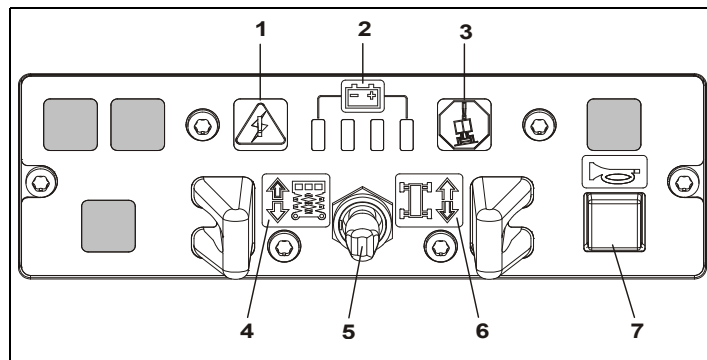
Fig. 3-8. Plattformsreglage/varningslampor
