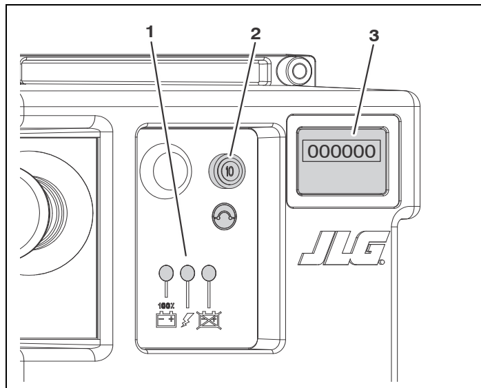
Fig. 3-4. Batteriladdningslampor/timmätare
